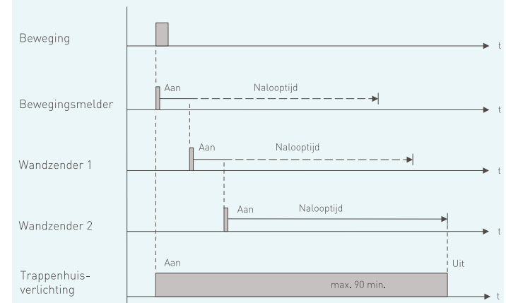
Werkingsprincipe trappenhuisverlichtingsschakeling
