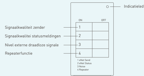
eNet diagnose-apparaat
